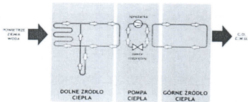
Rysunek 17 Zasada działania pompy ciepła,
