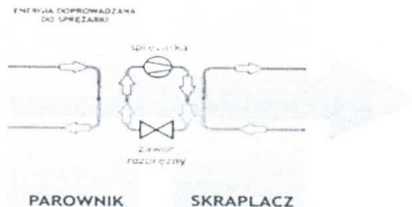
Rysunek 18 Obieg pośredni pompy ciepła,
