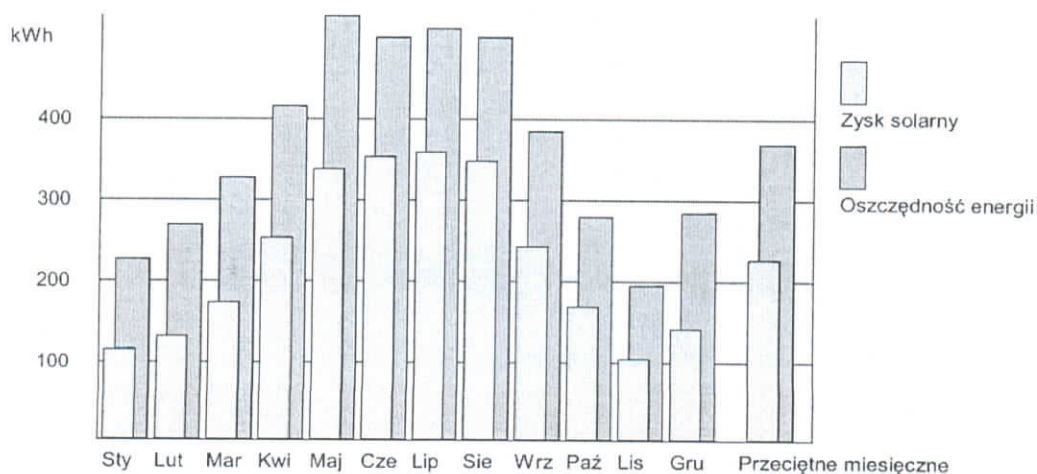
Rysunek 13 Symulacja wykorzystania kolektorów słonecznych, jako wspomaganie układu c.w.u. dla wspomaganie kotła węglowego,
